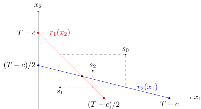
Figura 11: Grafico delle risposte r_1(x_2) e r_2(x_1) , e primi tre passi del metodo MRS
